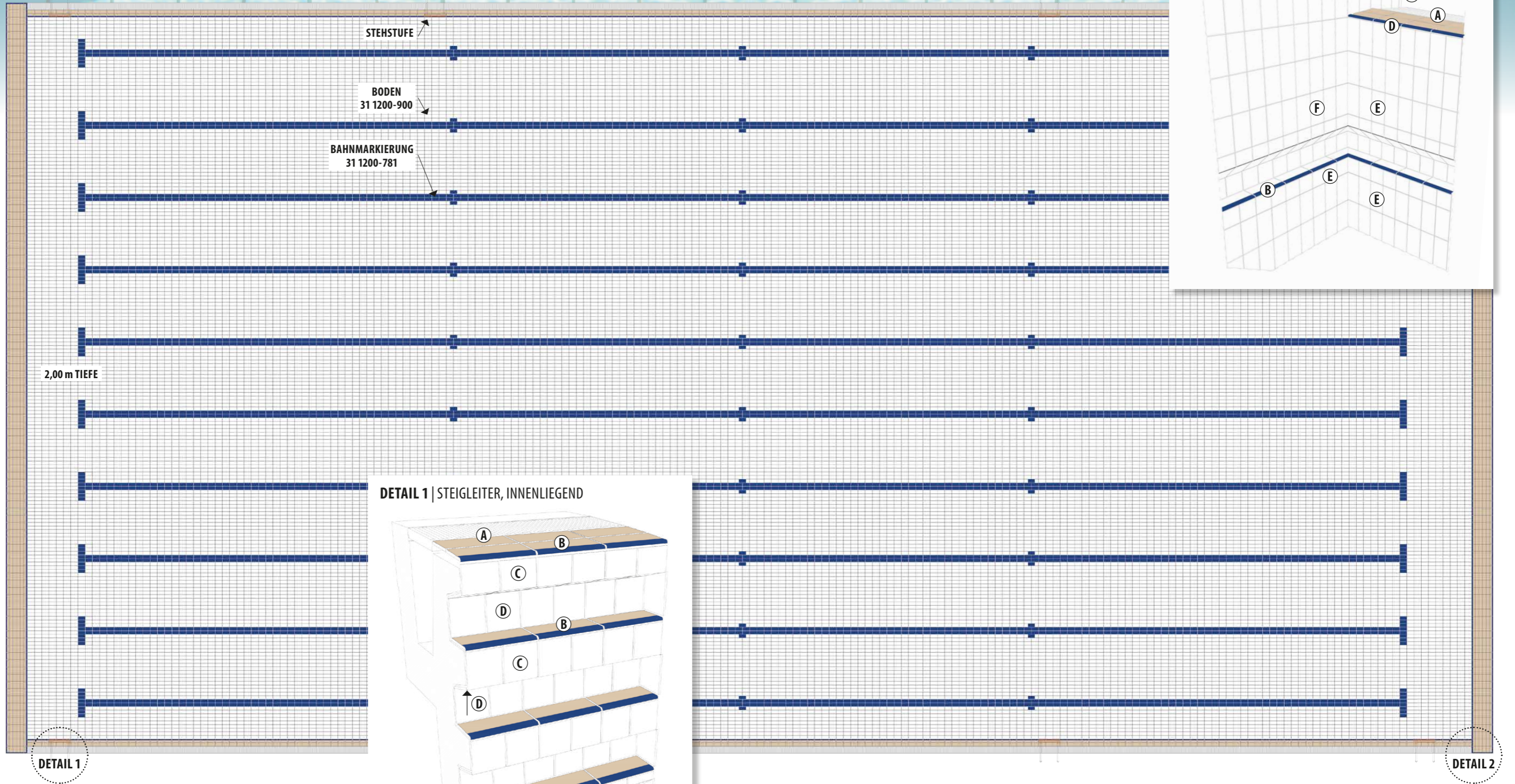
Artikelübersicht Detail 1 | Steigleiter, innenliegend
