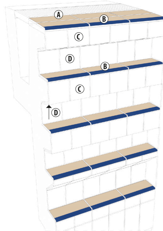
DETAIL 1 | STEIGLEITER, INNENLIEGEND
